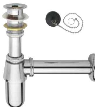
266010540 IT_ A bottiglia tipo tedesco 1"1/4 con piletta EN_ Bottle trap 1"1/4, german type with waste FR_ Siphon PVC 1"1/4 lavabo avec vidage GR_ σιφώνι χρωμέ με βαλβίδα
