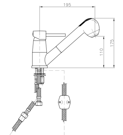
MIO28 IT_ Monocomando lavello, doccia estraibile 2 getti EN_ Sink mixer, twin-jet hand shower FR_ Mitigeur évier monotrou avec douchette jet double GR_ αναμεικτική μπataρια πiαγκου νεροχυτή με αποσπiσιμο ρουζουνι
