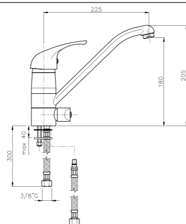
12122 IT_ Monocomando lavello, attacco lavastoviglie EN_ Sink mixer, dishwashing machine connection FR_ Mitigeur évier bec mobile, avec branchement pour machine à laver GR_ μπαταρία νεροχυτη με δυνατοτητα συνδεσης σε πλυντήριο πιάτων
