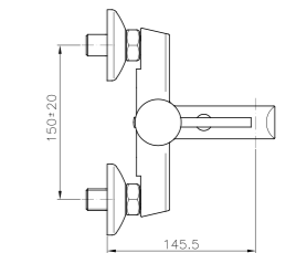
MI056 IT_ Monocomando vasca esterno senza duplex EN_ Bath mixer without duplex shower set FR_ Mitigeur bain-douche mural sans ensemble douche GR_ Επτοιχία αναμεικτική μπασίνα λουτρού, χωρίς τηλεφωνό σπιραλ και στρίγμα
